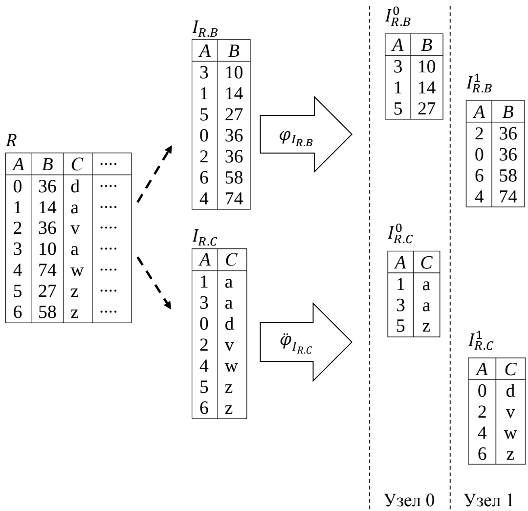
Рис. 6. Транзитивная фрагментация.
