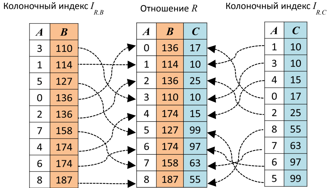
Рис. 4. Колоночные индексы.
